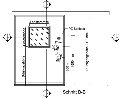
Rohbaumaß 1510 mm Zargenlichtmaß 1470 mm Freier Durchgang 1345 mm Türeinstand 125 mm
