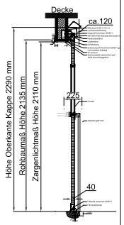
Schnitt A-A
