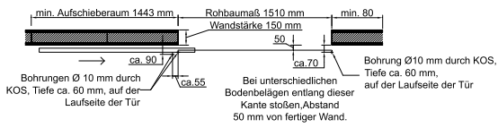
Schnitt E-E
